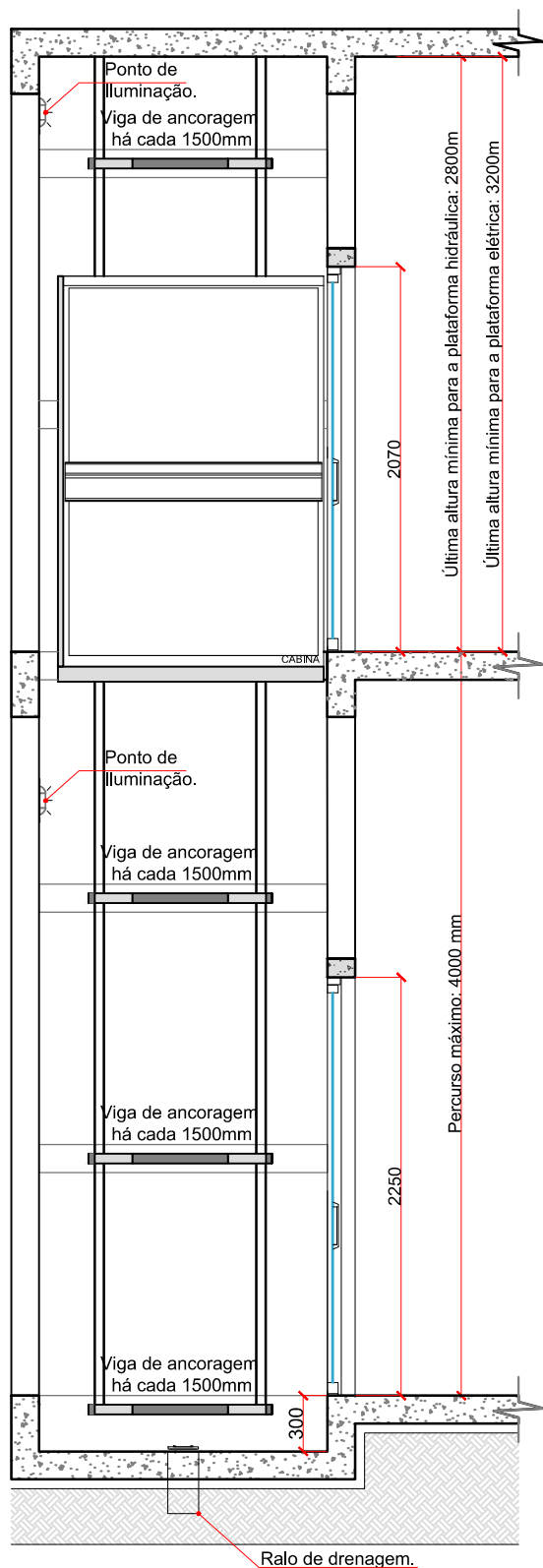
CORTE ESQUEMÁTICO
